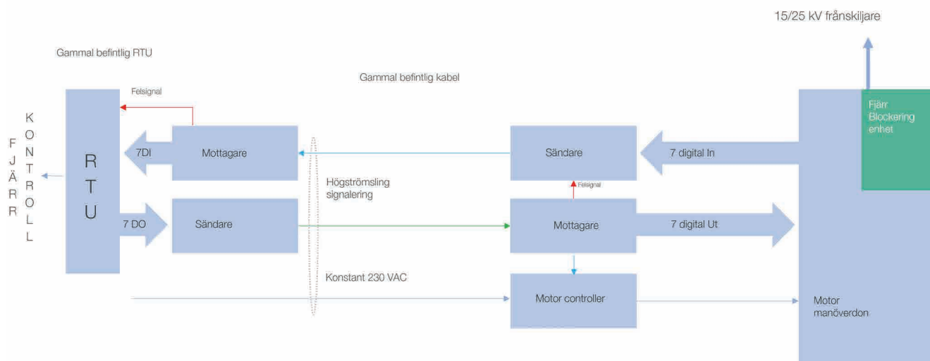
Funktionsprincip
